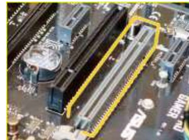
PCIe x16
